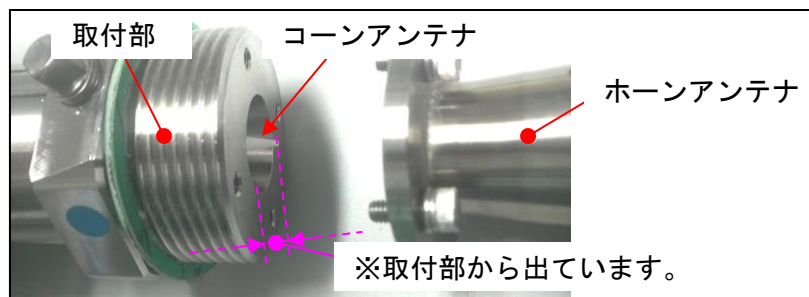
第9図. ホーンアンテナを取外した状態
