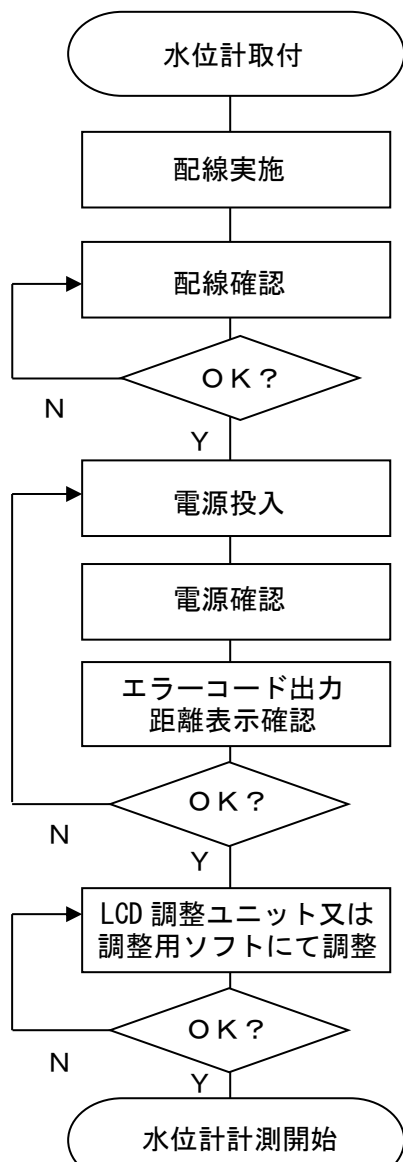
第 14 図. スタートアップフロー
