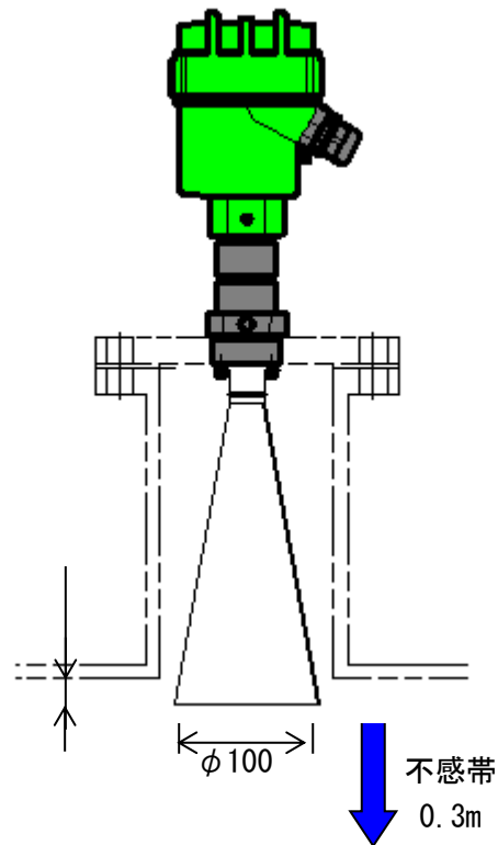
第4図. 本体取付
