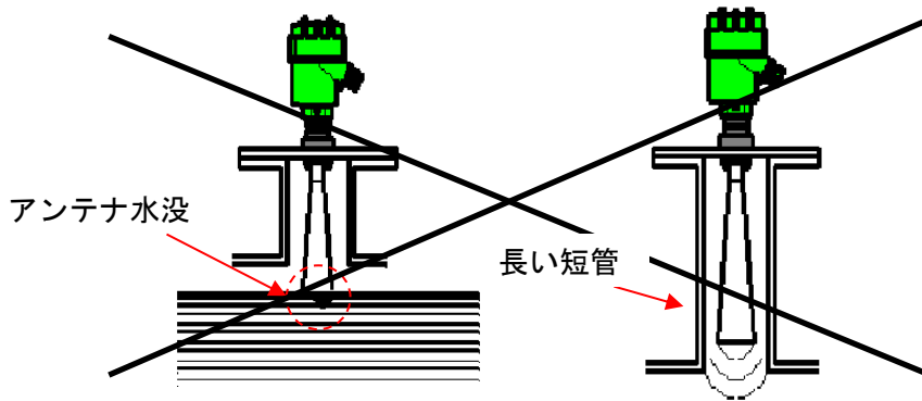
第7図. 取付上の注意 (その1)
