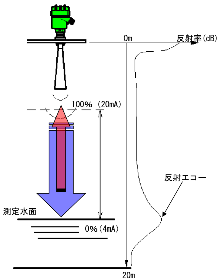
第 15 図. 計測イメージ
