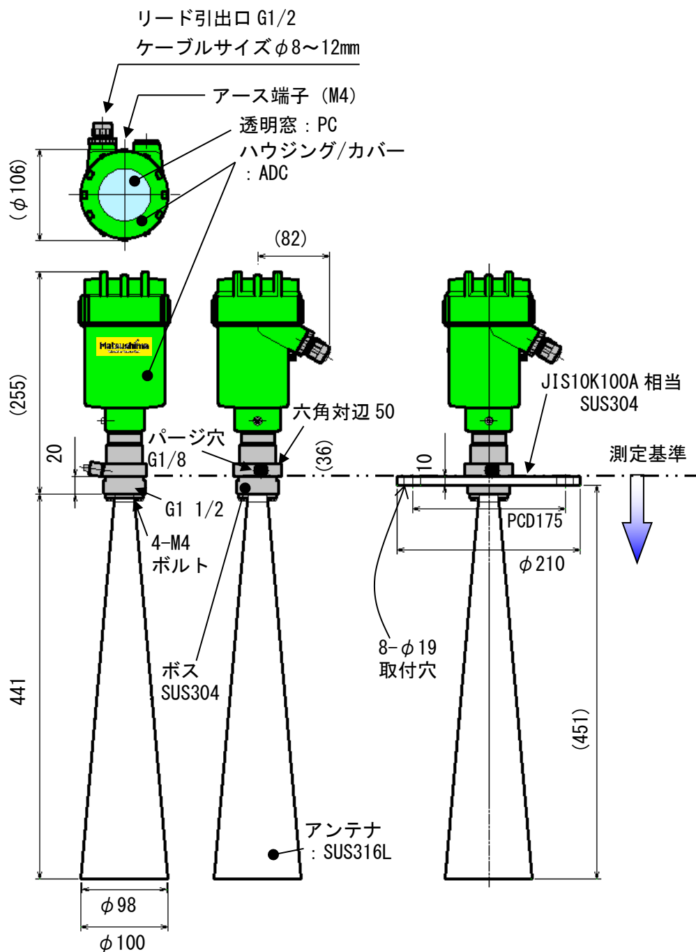
第3図. 水位計の外形
