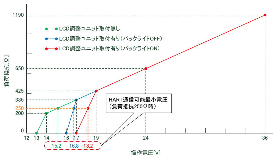
第 1 図. 操作電源と負荷抵抗
