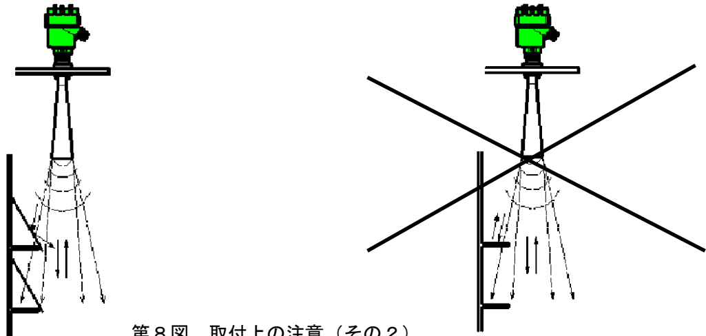
第8図. 取付上の注意（その2）
