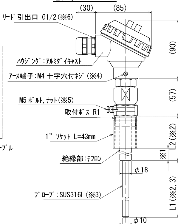
センサ : PFM-M11P
