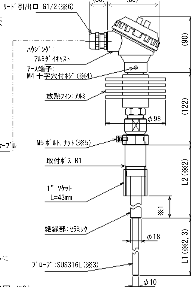
第2図 外形図 (略)
