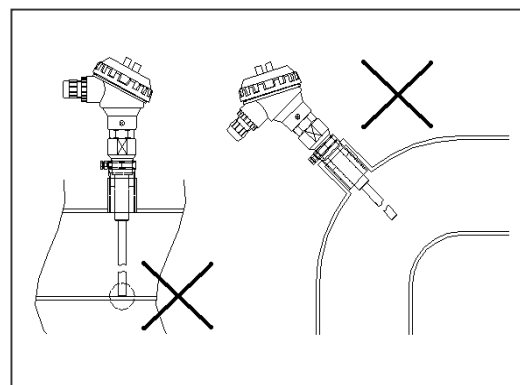
第4図 良くない取付例
