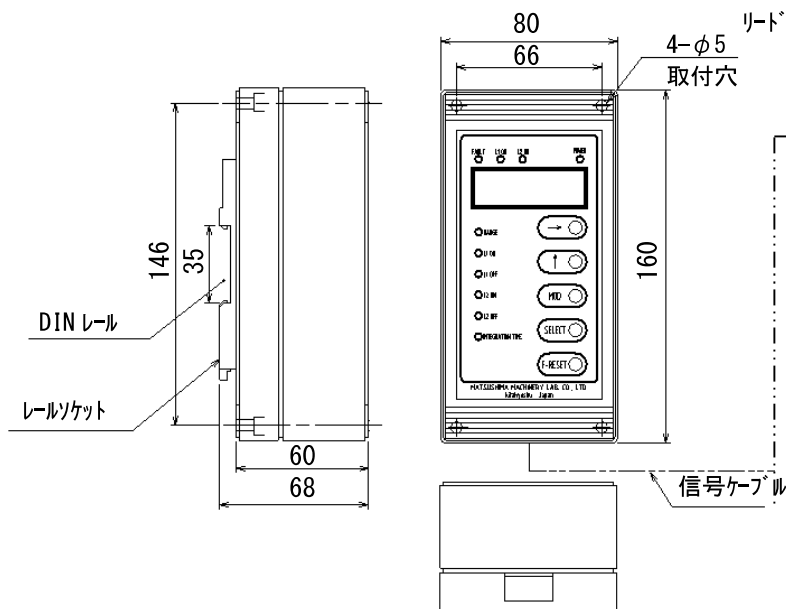
変換器 : PFM-KCU11
