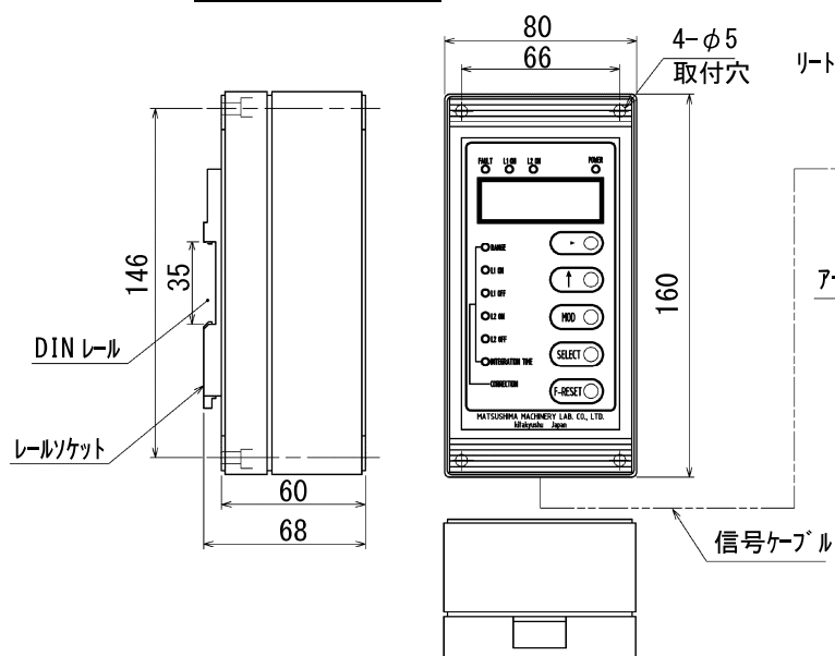
変換器 : PFM-KCU11
