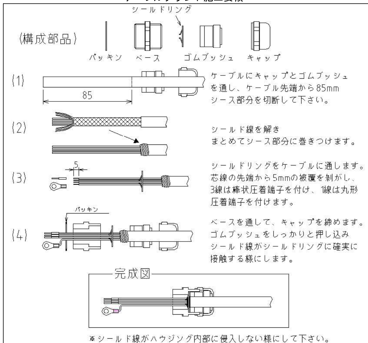
第11図 ケーブル施工要領
