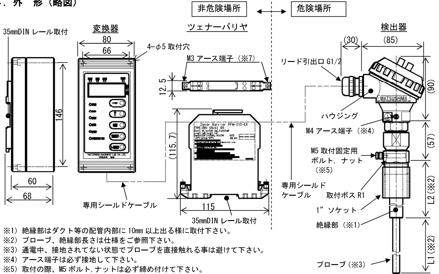
第3図 外形図（略）
