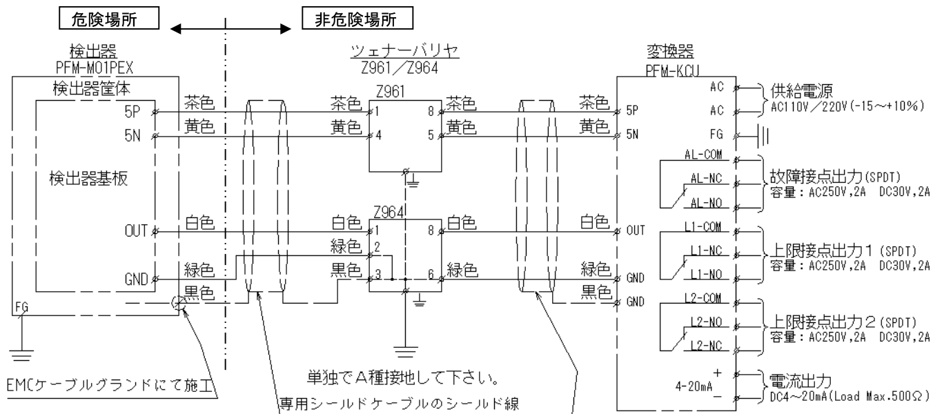
第10図 接続図
