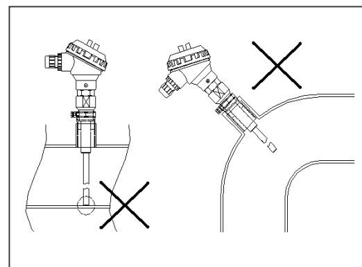
第5図 良くない取付例
