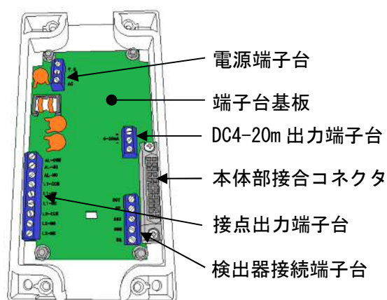
第8図 端子台部
