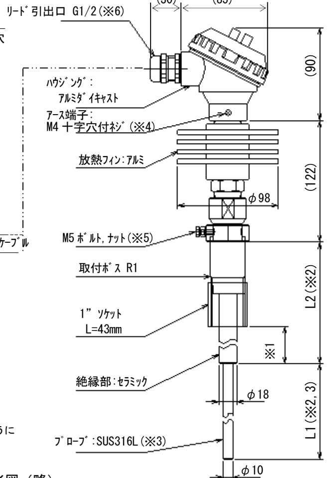
第2図 外形図 (略)
