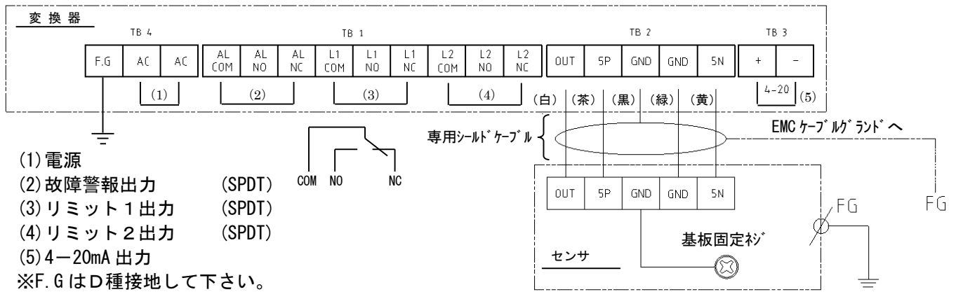
第 9 図 接続図
