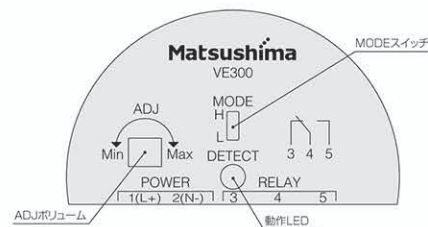
端子台部
