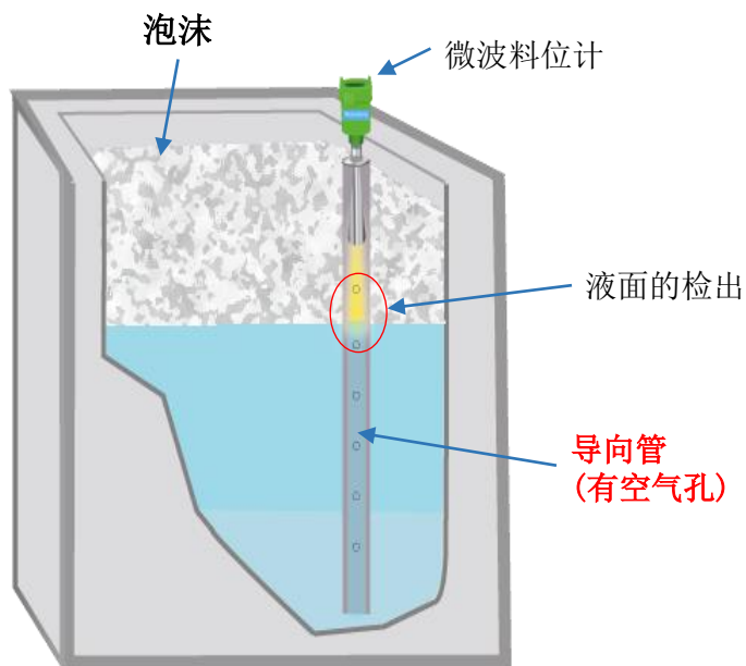
※图以及照片：导向管内无泡沫检出液面的样子
